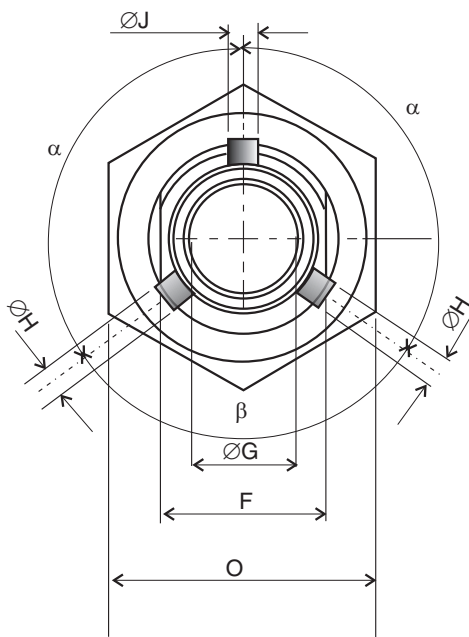
3 Lug Version
