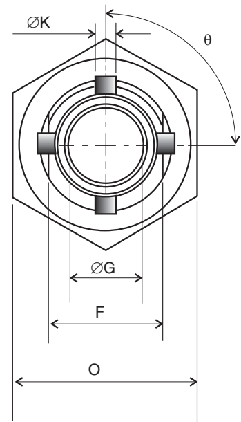
4 Lug Version
